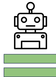
Algoritmo
